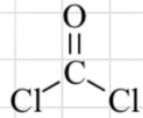
fosgênio
