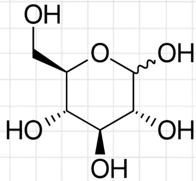
glicose
