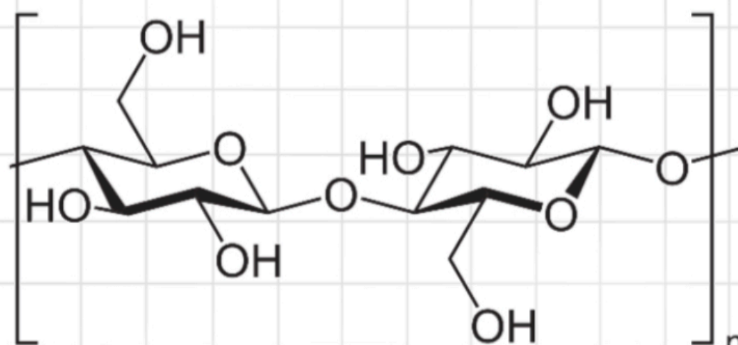
celulose
