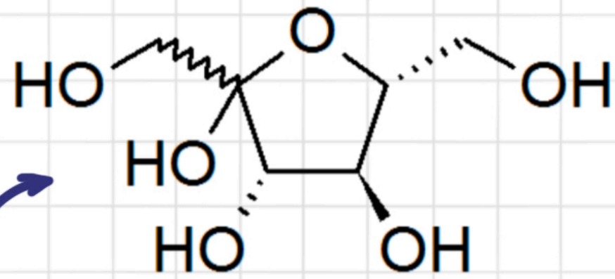
frutose
