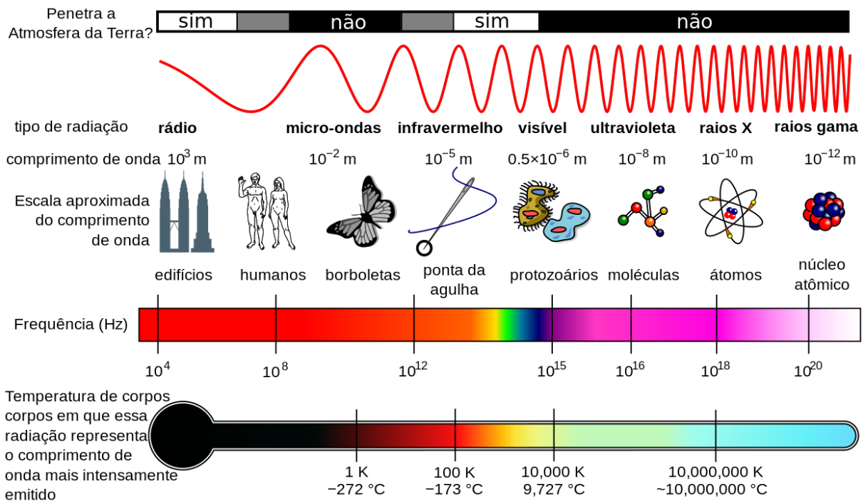
Espectro Eletromagnético
