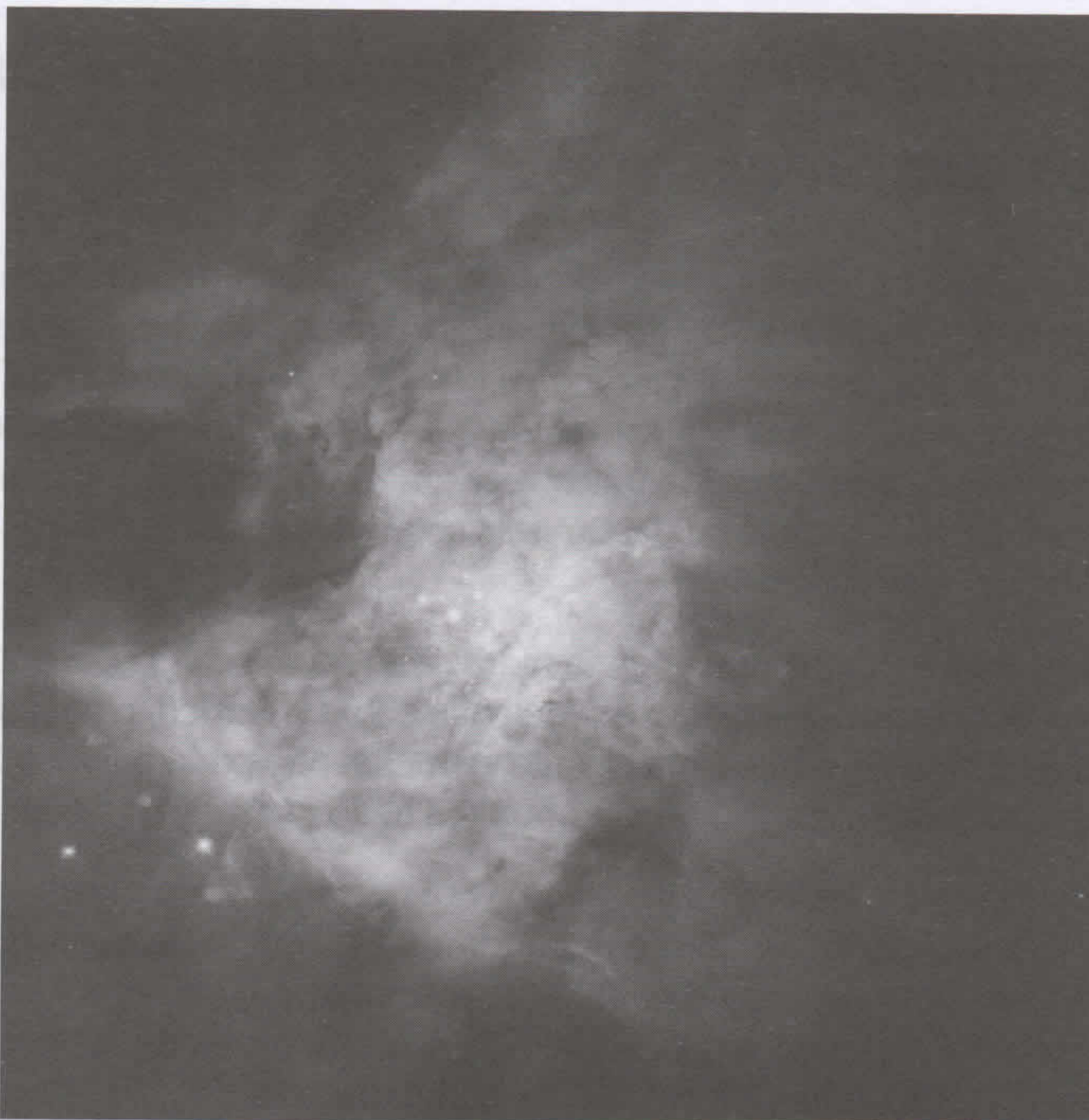
Figura 11-1: A nebulosa de Orion hospeda muitos objetos estelares jovens.
