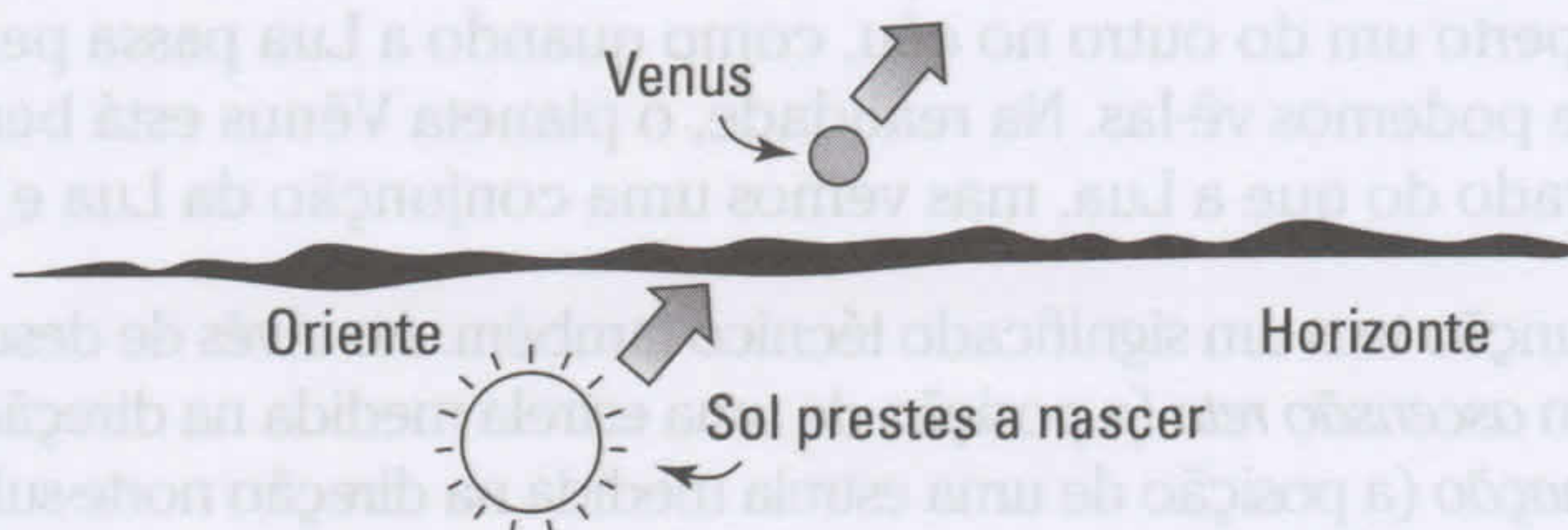
Vênus como Estrela da Manhã
