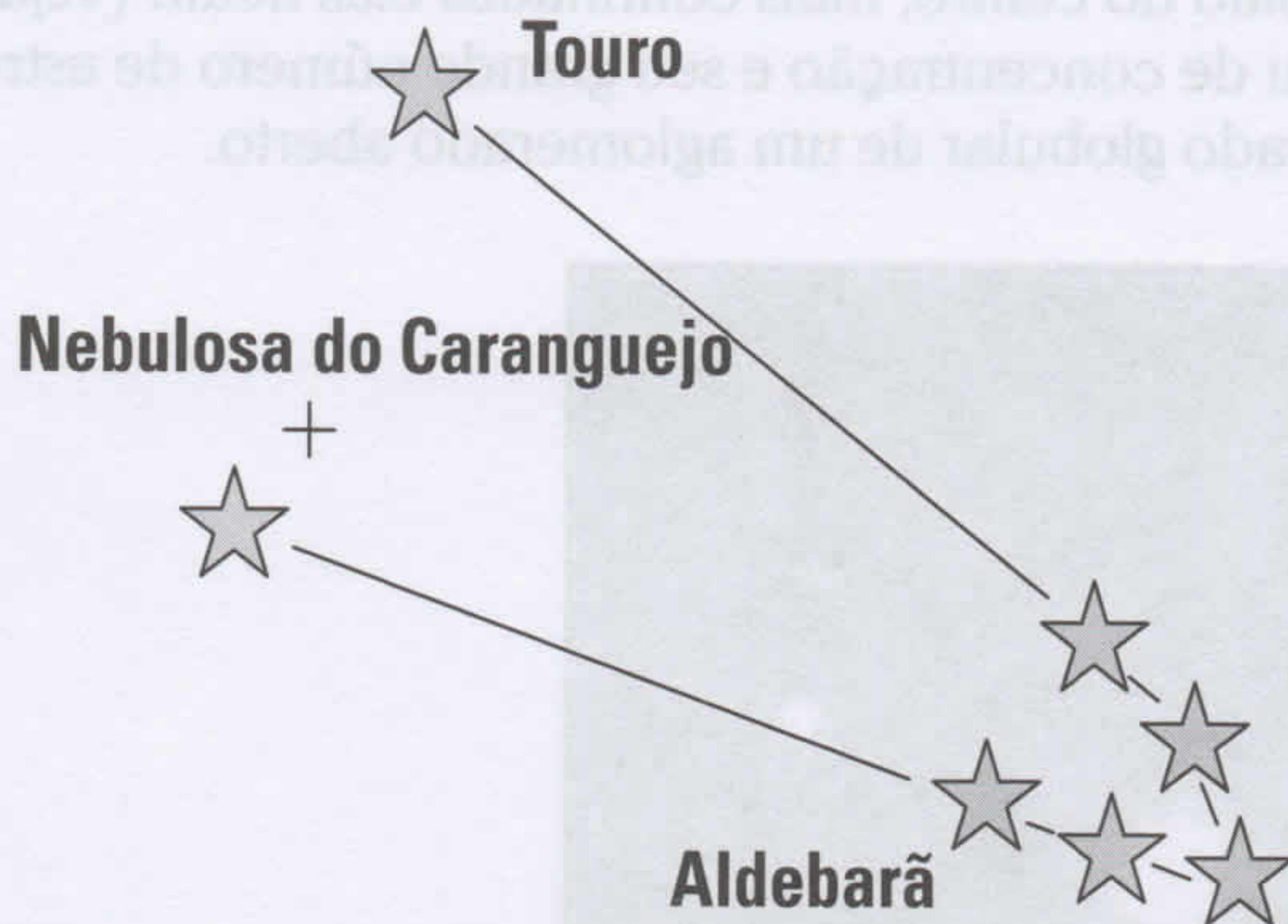
Figura 12-2: Touro contém a gigante vermelha Aldebarã (Alpha Tauri).
