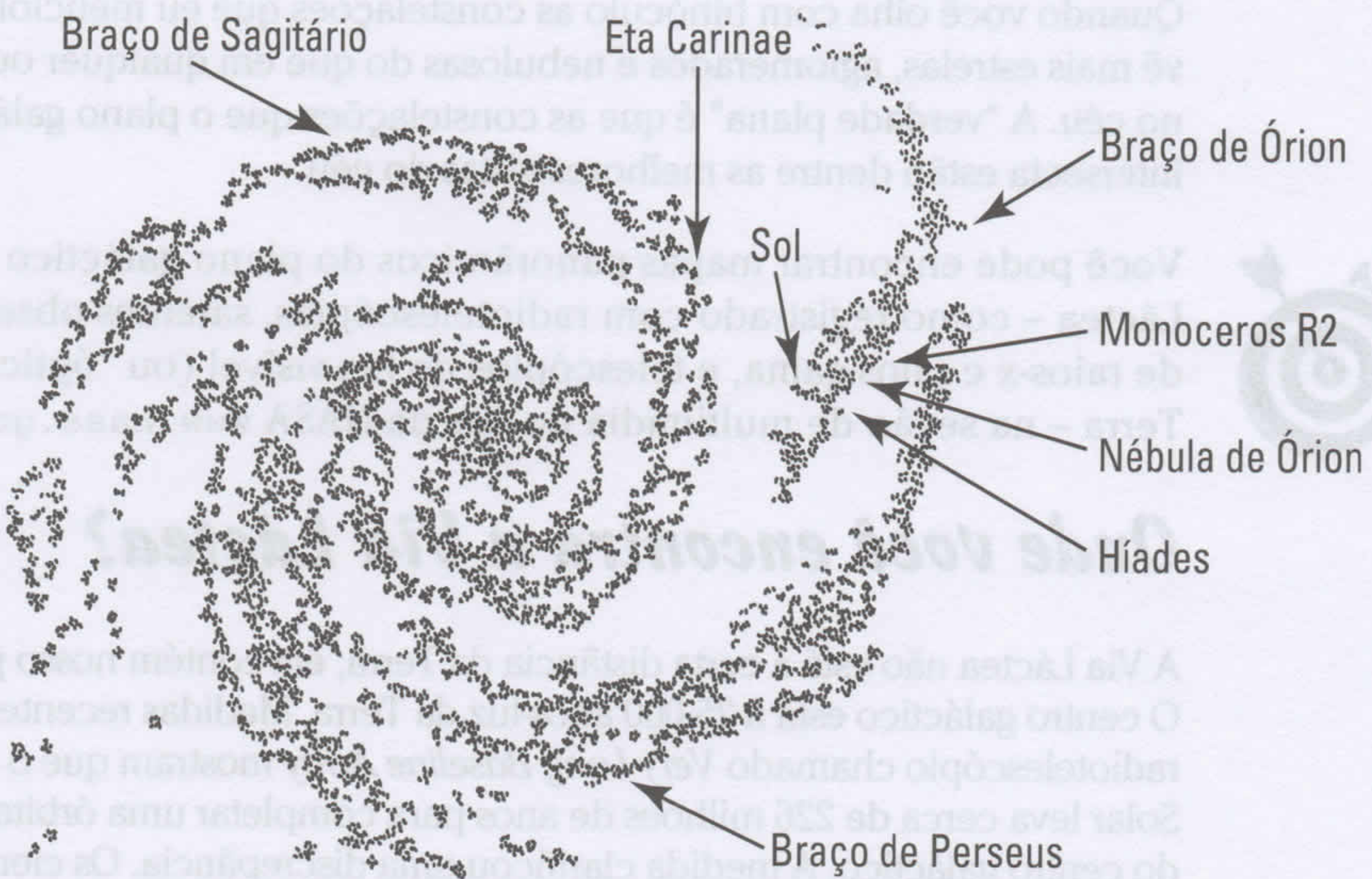
Figura 12.1: A Via Láctea é uma galáxia espiral com braços rodeando o centro galáctico.
