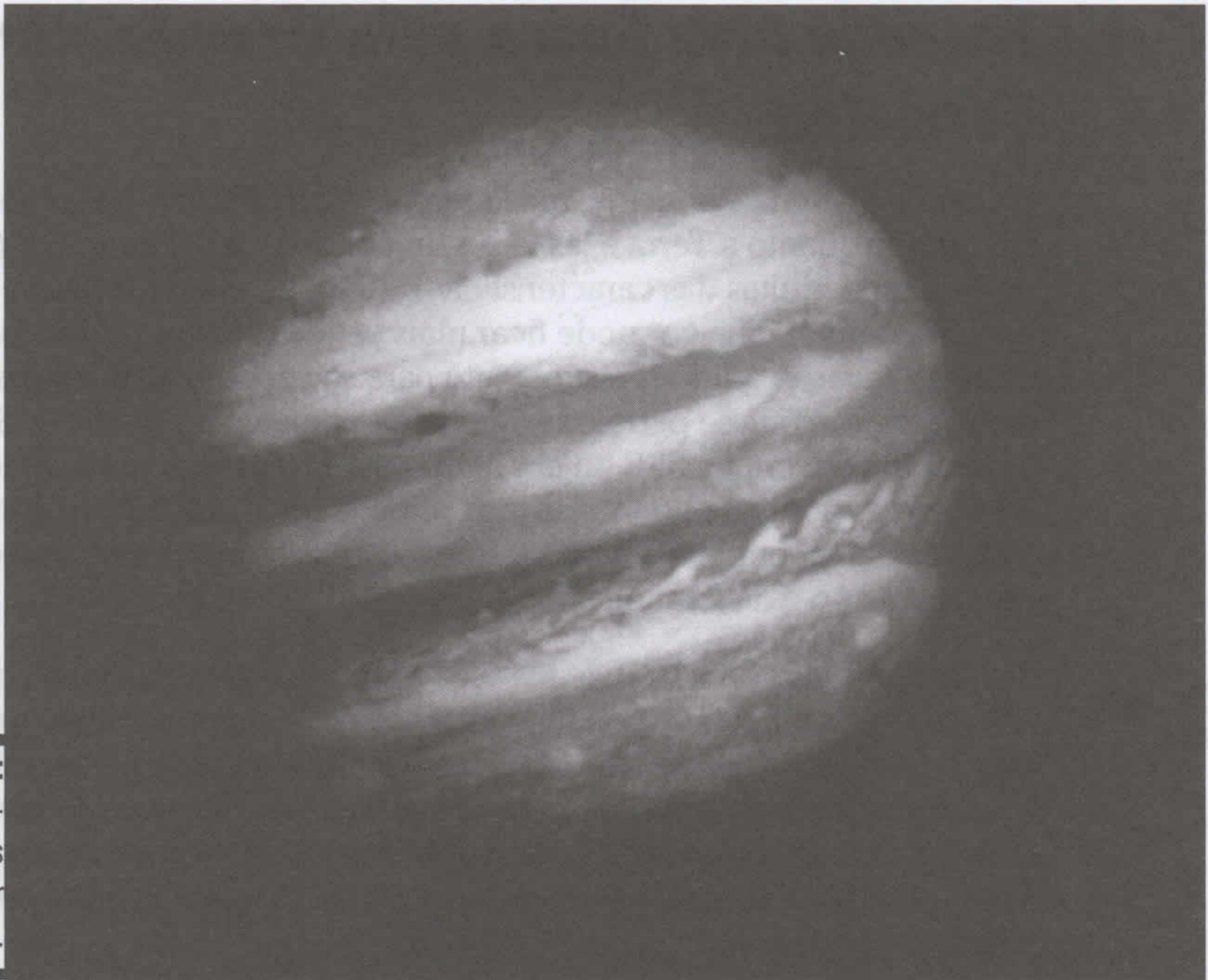
Figura 8-1: Júpiter e as faixas de nuvens induzidas por sua rotação.
