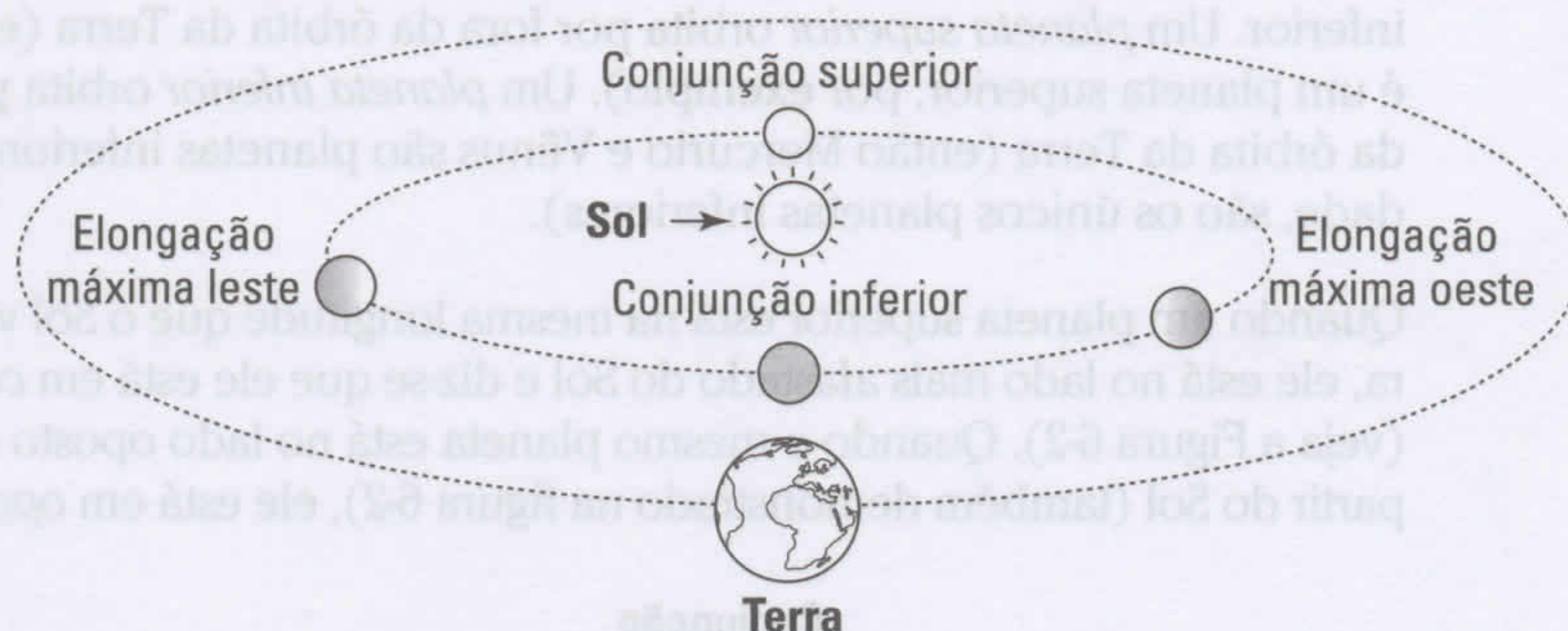
Figura 6-3: A conjunção inferior se alinha a um planeta inferior com o Sol na direção leste-oeste.
