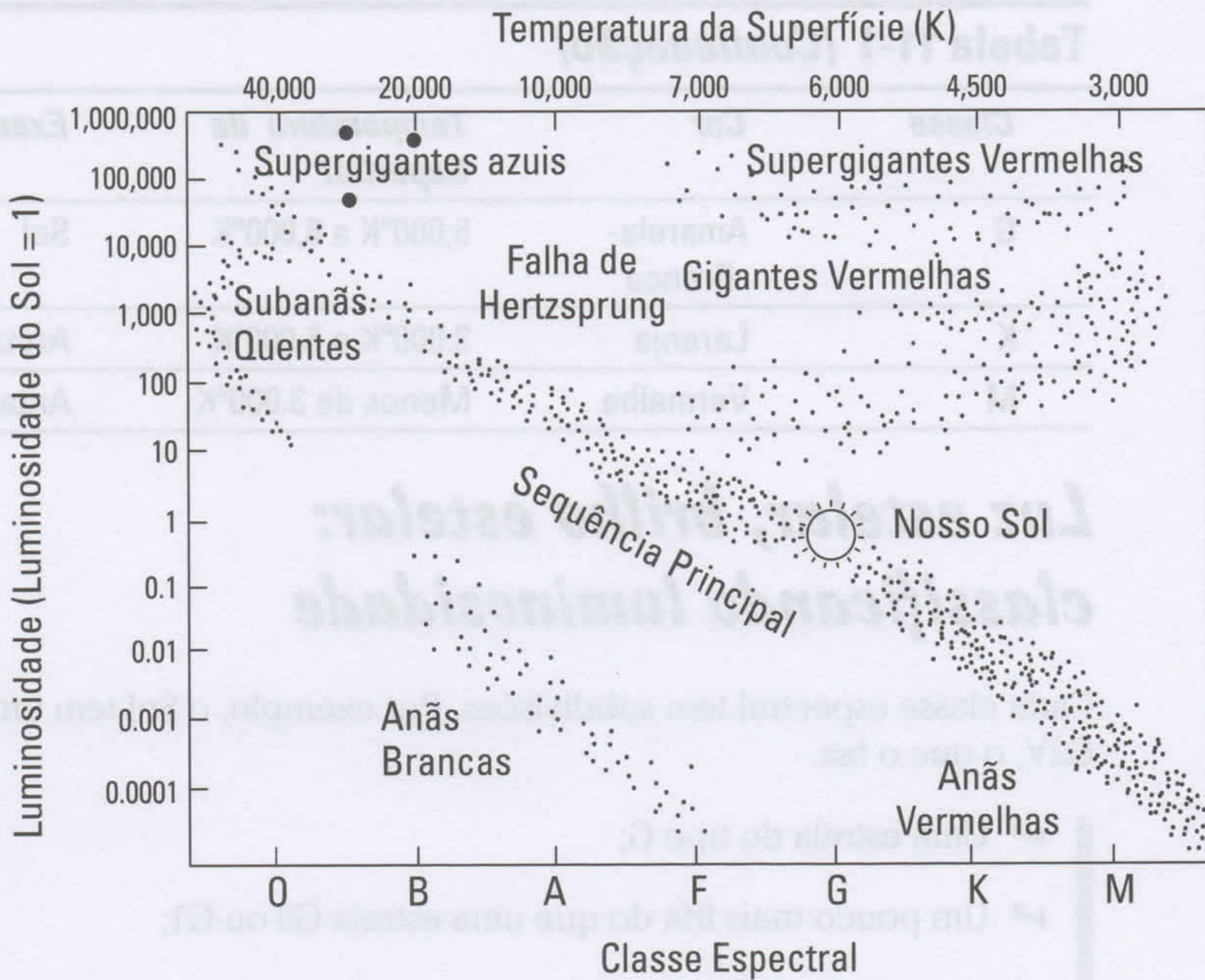
Figura 11-4: O diagrama Hertzsprung-Russell mostra o brilho e a temperatura das estrelas.
