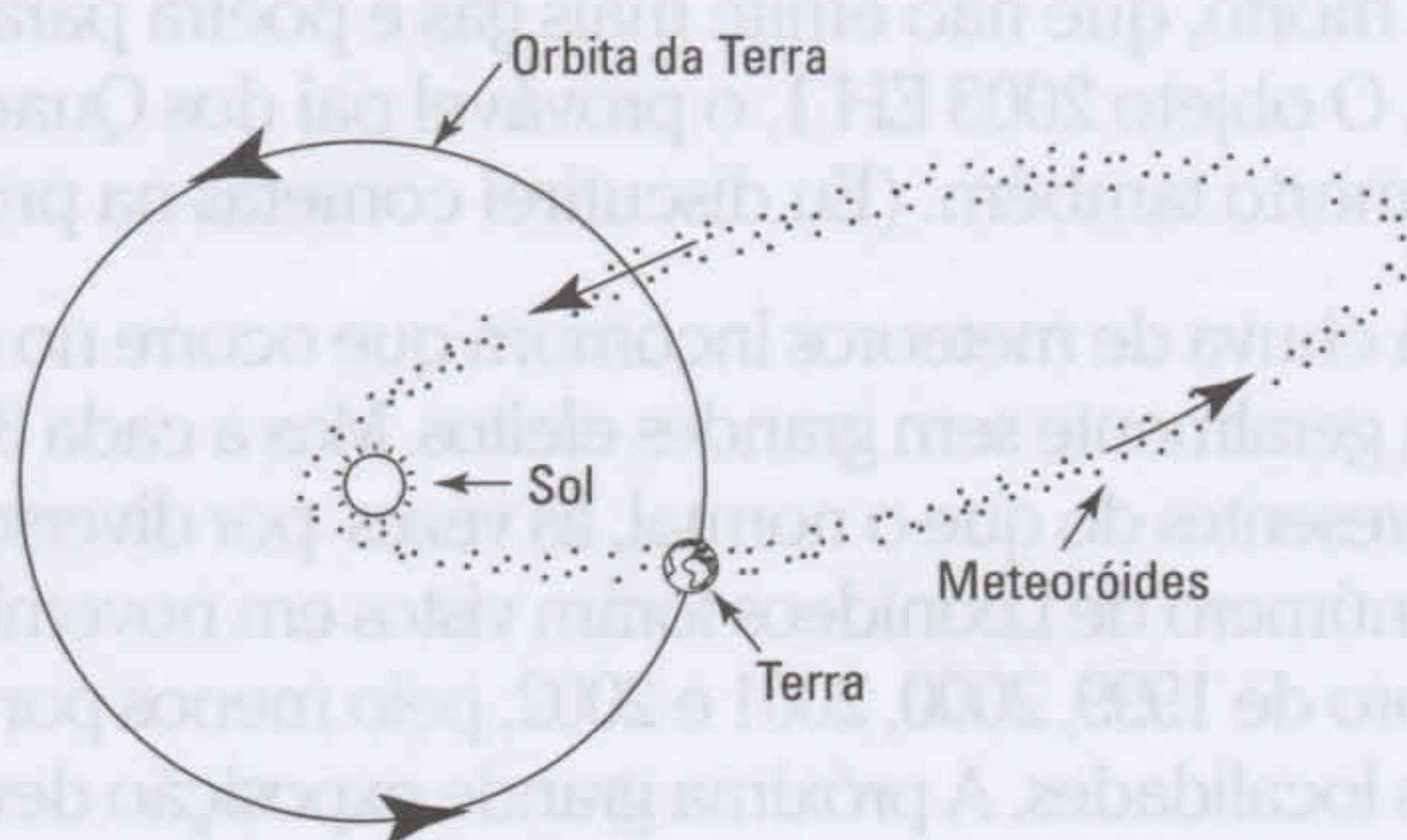
Figura 4-1: O caminho da Terra cruzando um cinturão de meteoróides cria uma chuva de meteoros.
