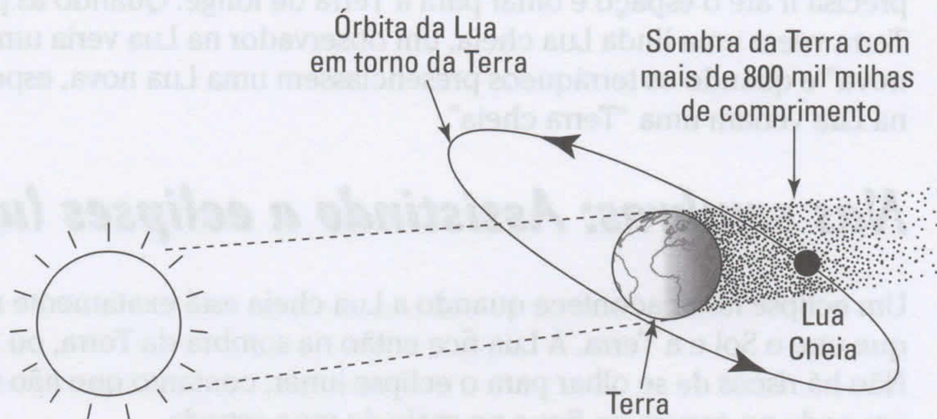
Figura 5-5: Um eclipse total da Lua.
