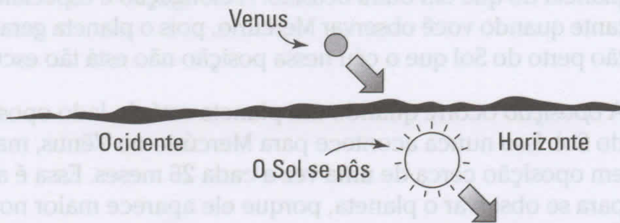
Vênus como Estrela Vespertina
