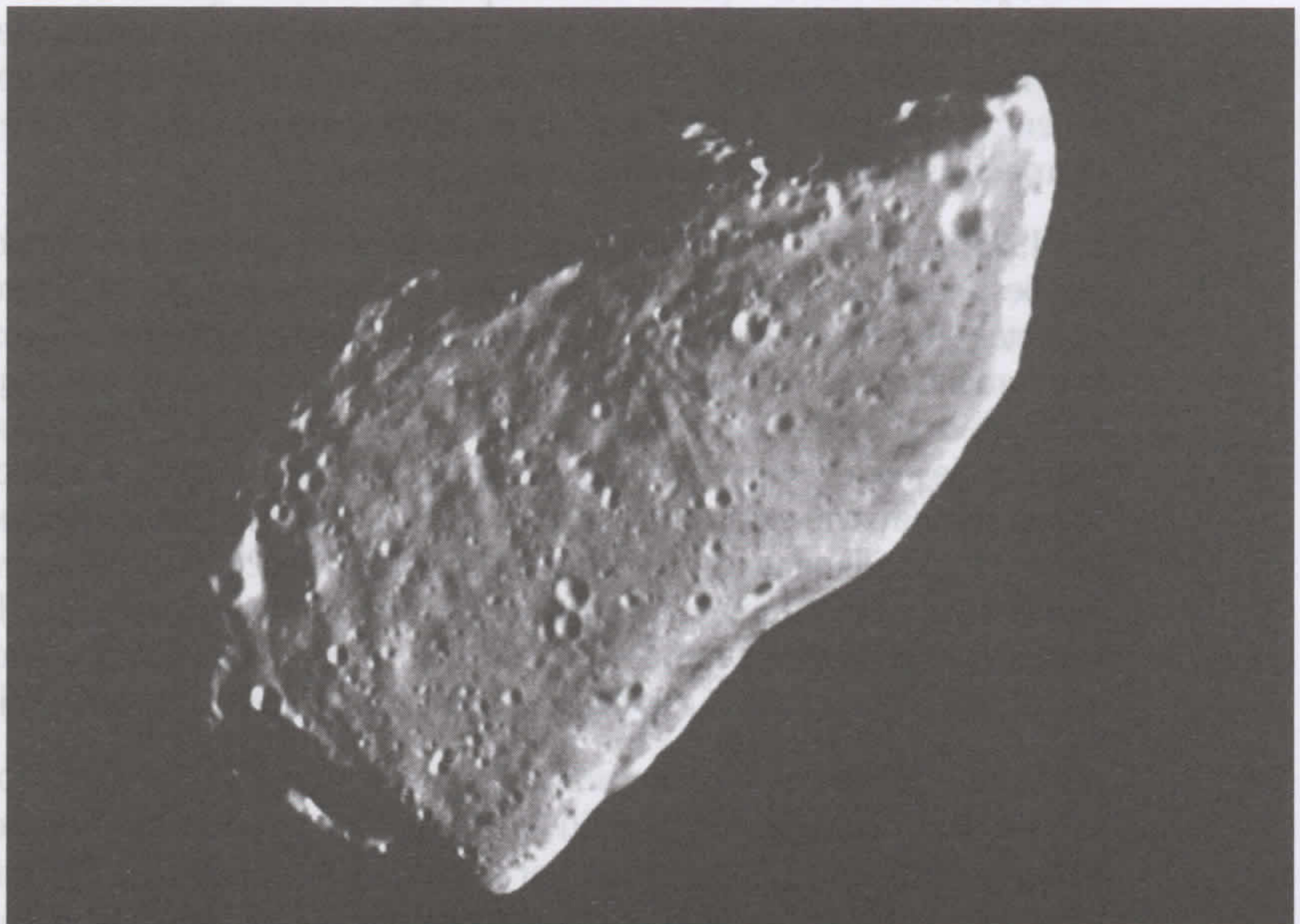
Figura 7-2: Alguns asteroides parecem grandes batatas.
