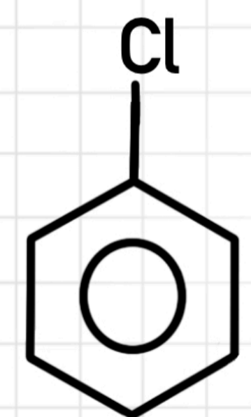
Clorobenzeno ou Cloreto de fenila
