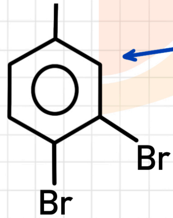
1,2-dibromo-4-metilbenzeno
