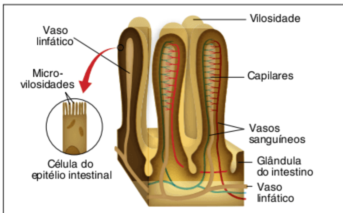
Fig. 10 Estrutura de vilosidades intestinais.
