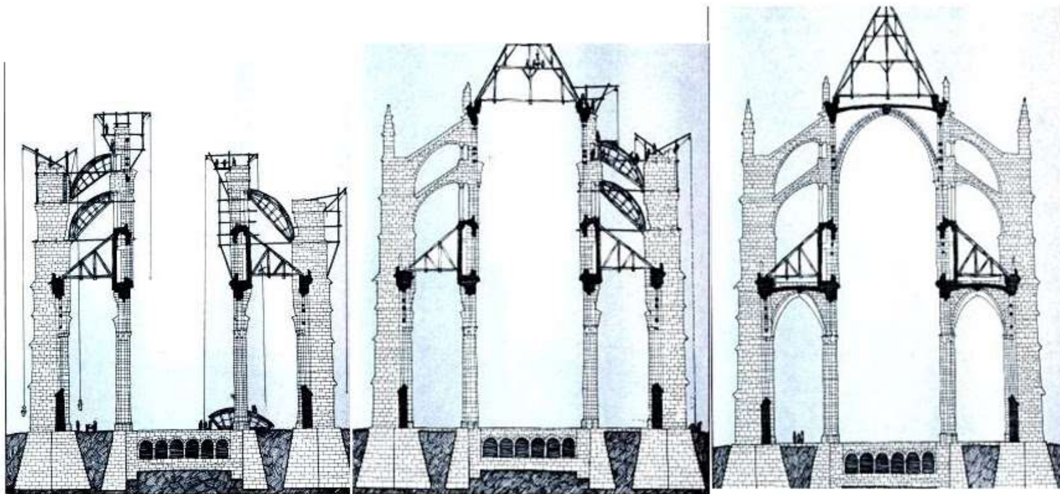
Sistema de construção de uma catedral gótica
