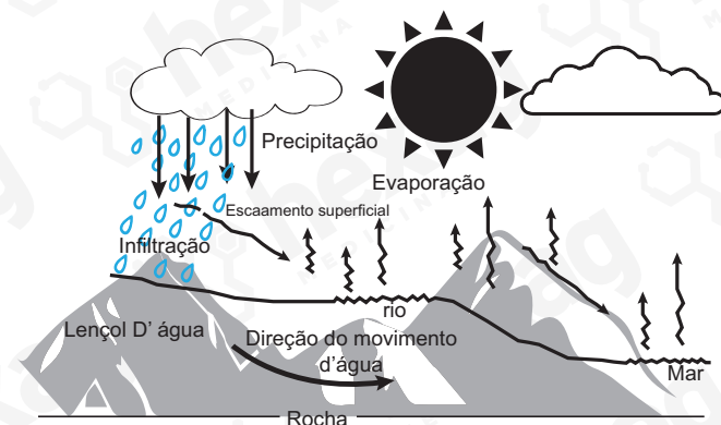
Esquema representa o ciclo hidrológico. Fonte: Adaptado de Silva Filho (1998).
